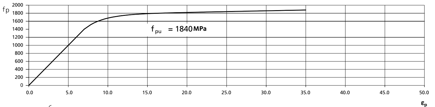
Acero para pretensado C-1900 en cordones de siete alambres baja relajación Gráfica f_p - \epsilon_p
